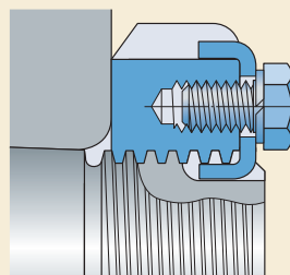
Trava com presilha
