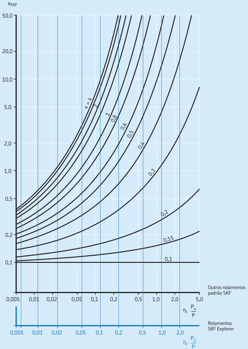
Fator a_{SKF} para rolamentos de esferas radiais
