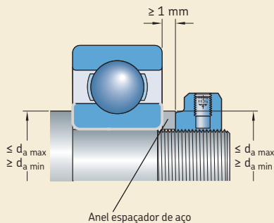
Anel espaçador de aço
