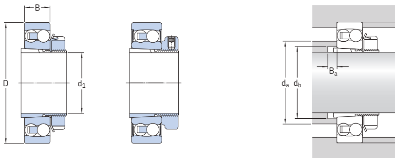
Rolamento aberto em uma bucha modelo E
