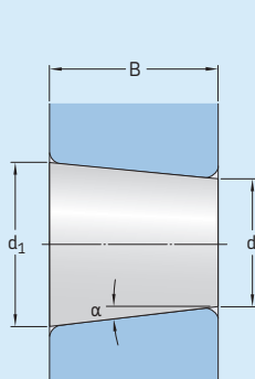
Tolerâncias Normais para furos cônicos, conicidade 1:30
