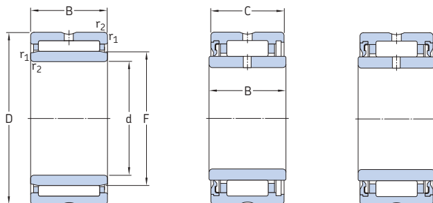
NKI(S) NA 49 NA 69
