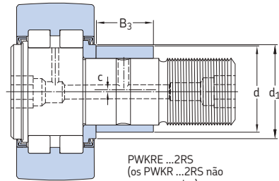
O rolo de leva com eixo A (NUKRE .. A possui um colar excêntrico)
